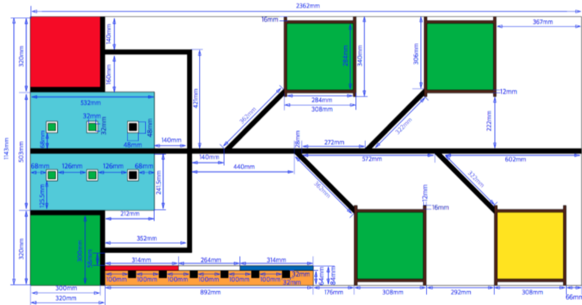
Figura 1. Especificaciones técnicas de la pista de acuerdo a la WRO llevada a cabo en el 2017 para la categoría de secundaria.
