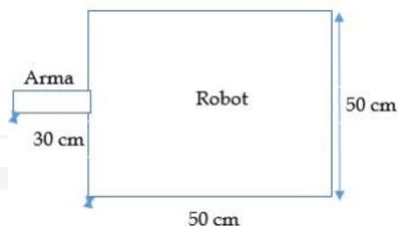
Figura 1. Dimensiones del robot
